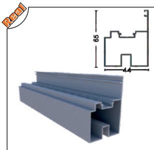
PRGLD-1008 8 mm İspanyollet Kol Profili 8 mm Espagnolette Arm Profile
