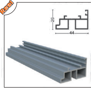
PRGLD-1006 Tıjlı Kollu Fitil Karşılığı Espagnolette Arm Opposite Seal
