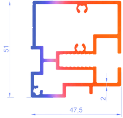
T.2480 -1,459 KG/MT HAREKETLİ DİKME PROFİLİ
