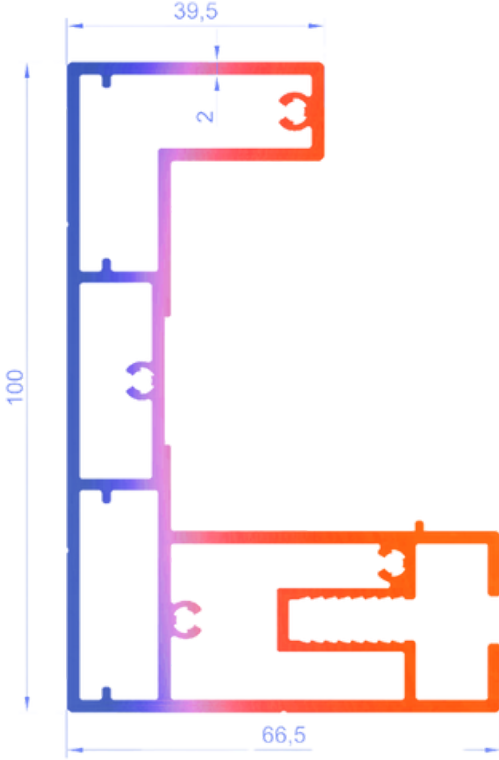
T.2479- 2,718 KG/MT SABİT DİKME PROFİLİ
