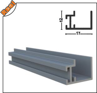
SRM-1010 Çekme Profili (10 mm) Pull Profile (10 mm)
