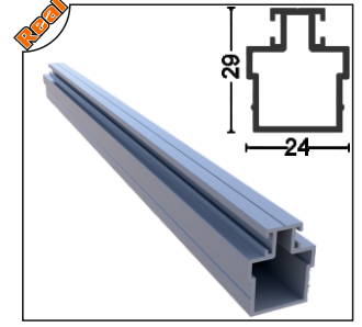
OPT-1015-50 Orta Birleşim Profili Middle Joint Profile
