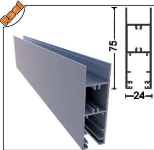
OPT-1010-60 Baza Profili Isıcamlı Glass Profile Double Glazed Ağırlık/Weight 0.968 kg/m
