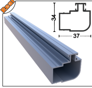
OPT-1016-50 90° Birleşim Profili 90° Joint Profile
