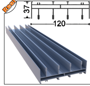
OPT-1005-60 Üst Kasa 4 Raylı Upper Frame Profile 4 Rails Ağırlık/Weight 1.855 kg/m
