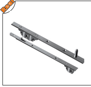
OPT-2016 Sürme İspanyolet 180 cm Slide Espagnolette 180cm
