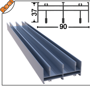
OPT-1002-60 Üst Kasa 3 Raylı Upper Frame Profile 3 Rails Ağırlık/Weight 1.46 kg/m
