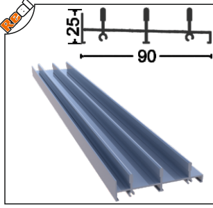
OPT-1001-60 Alt Kasa 3 Raylı Lower Frame Profile 3 Rails Ağırlık/Weight 1.06 kg/m
