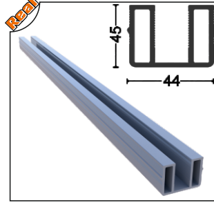
OPT-1017-60 8 mm Adaptör Profili 8mm Adapter Profile
