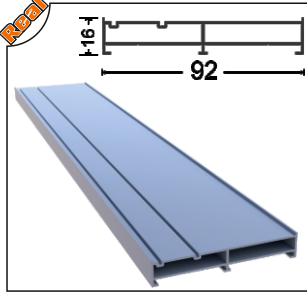
OPT-1003-50 Yan Dikme 3 Raylı Side Profile 3 Rails Ağırlık/Weight 0.886 kg/m
