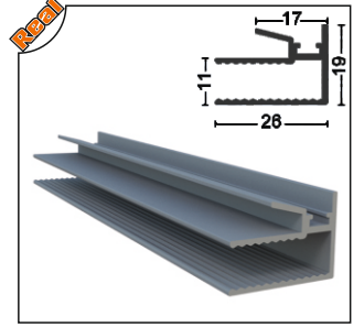
SRM-1009 Çekme Profili (8 mm) Pull Profile (8 mm)
