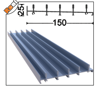
OPT-1007-60 Alt Kasa 5 Raylı Lower Frame Profile 5 Rails Ağırlık/Weight 1.68 kg/m
