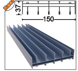
OPT-1008-60 Üst Kasa 5 Raylı Upper Frame Profile 5 Rails Ağırlık/Weight 2.246 kg/m
