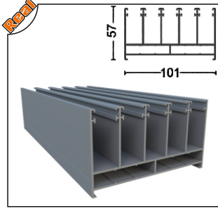
SRM-1001 Üst Kasa Profili Upper Frame Profile
