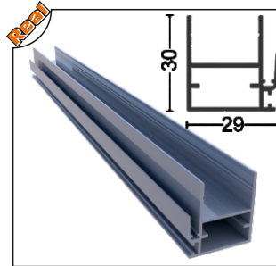
OPT-1011-50 Çekme Profili Isıcamlı Pull Profile Double Glazed Ağırlık/Weight 0.434 kg/m
