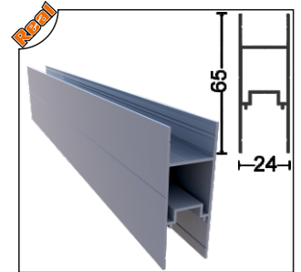
OPT-1012-50 İspanyolet Bitim Profil End Profile with Espagnolette Ağırlık/Weight 0.67 kg/m
