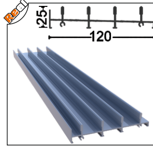
OPT-1004-60 Alt Kasa 4 Raylı Lower Frame Profile 4 Rails Ağırlık/Weight 1.37 kg/m
