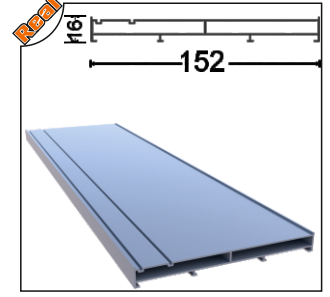
OPT-1009-50 Yan Dikme 5 Raylı Side Profile 5 Rails Ağırlık/Weight 1.35 kg/m
