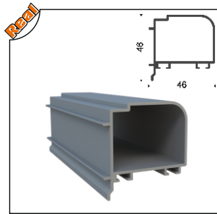
ISICM31-1014 90° Adaptör Aluminum 90° Seal
