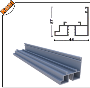
PRGLD-1009 İspanyolet Kol Profil Karşılığı 8 mm Espagnolette Arm Profile Of Opposite
